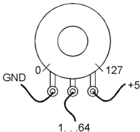
Anschluss eines Drehpotentiometers
